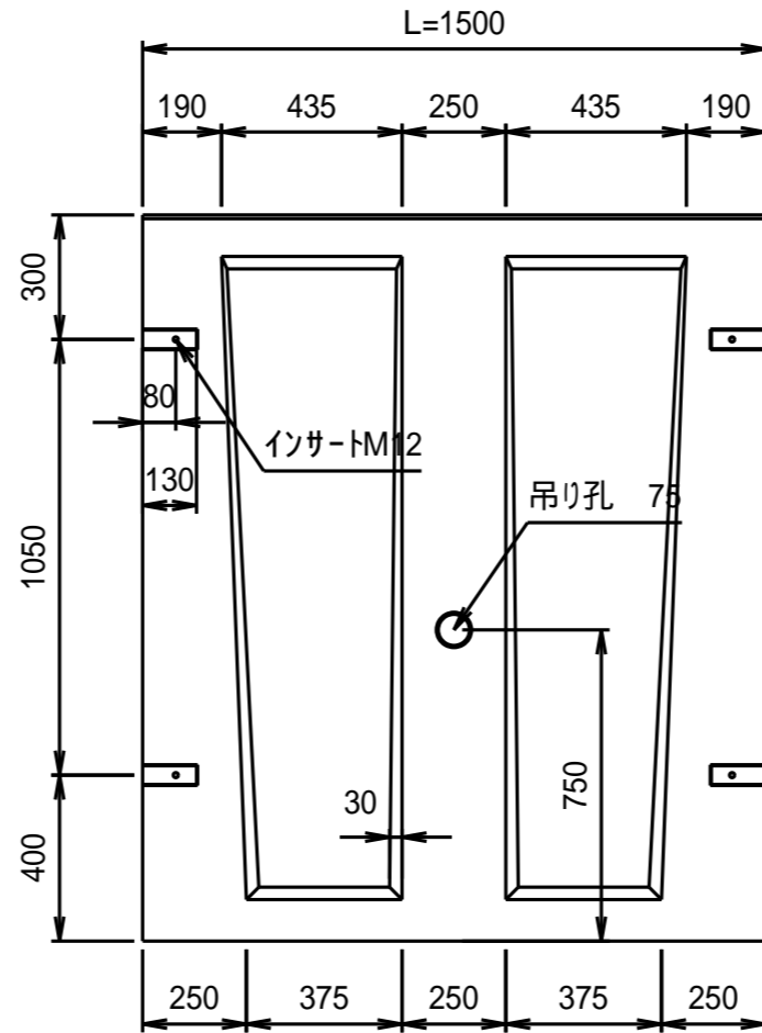
側面図
